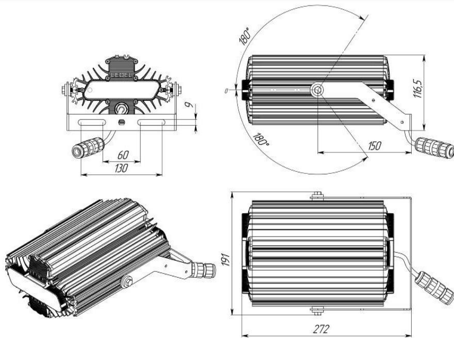
Рисунок 2 Светильник «L-lego 30 banner» Поворотное крепление
